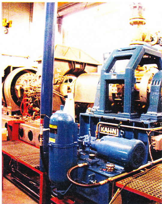
康氏108-130型号液力测力仪可在10000r/min速度下吸收12000kW，是丹麦皇家海军新建造的LM500发动机试验室的一个关键装置。
